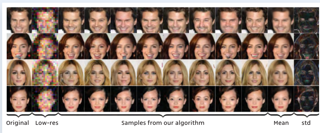
איור 4. פתרון בעיית סופר-רזולוציה (הגדלת תמונה נתונה) באמצעות מודלי דיפוזיה
