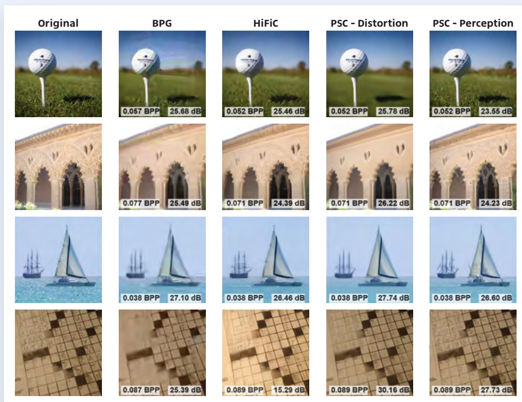
איור 5. תוצאות דחיסה-פריסה השוואתיות בין השיטה המוצעת ל-HiFiC
