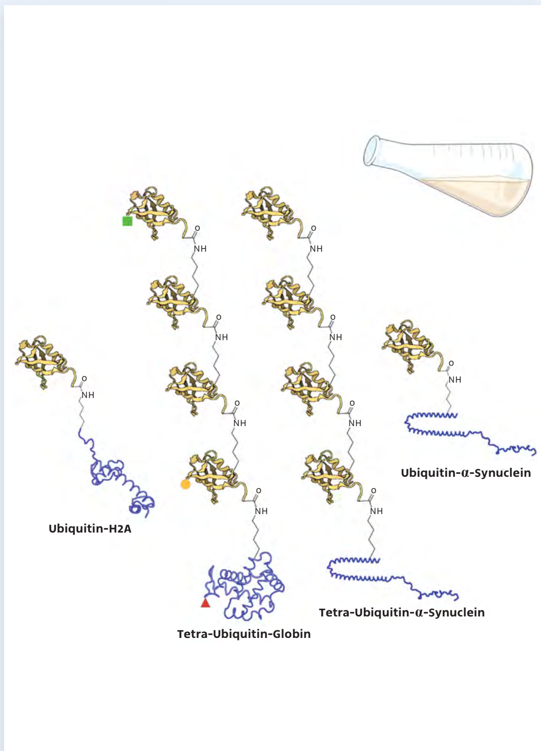
איור 3. סינתזה כימית של חלבונים מצומדים לאוביקוויטין ולשרשראות אוביקוויטין
