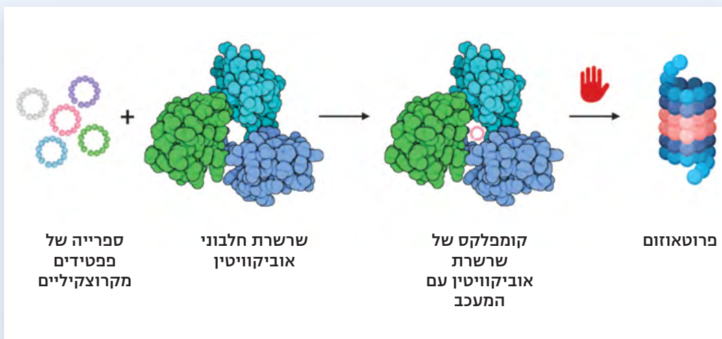
איור 4. עיכוב פירוק חלבונים מושג בעזרת פפטידים מקרוצקליים באמצעות קשירה לשרשרת האוביקוויטין
