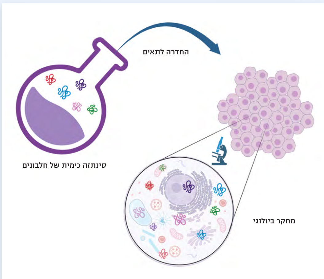
איור 5. סינתזה כימית של חלבונים מסומנים והחדרתם לתאים חיים למטרת מחקר ביולוגי
